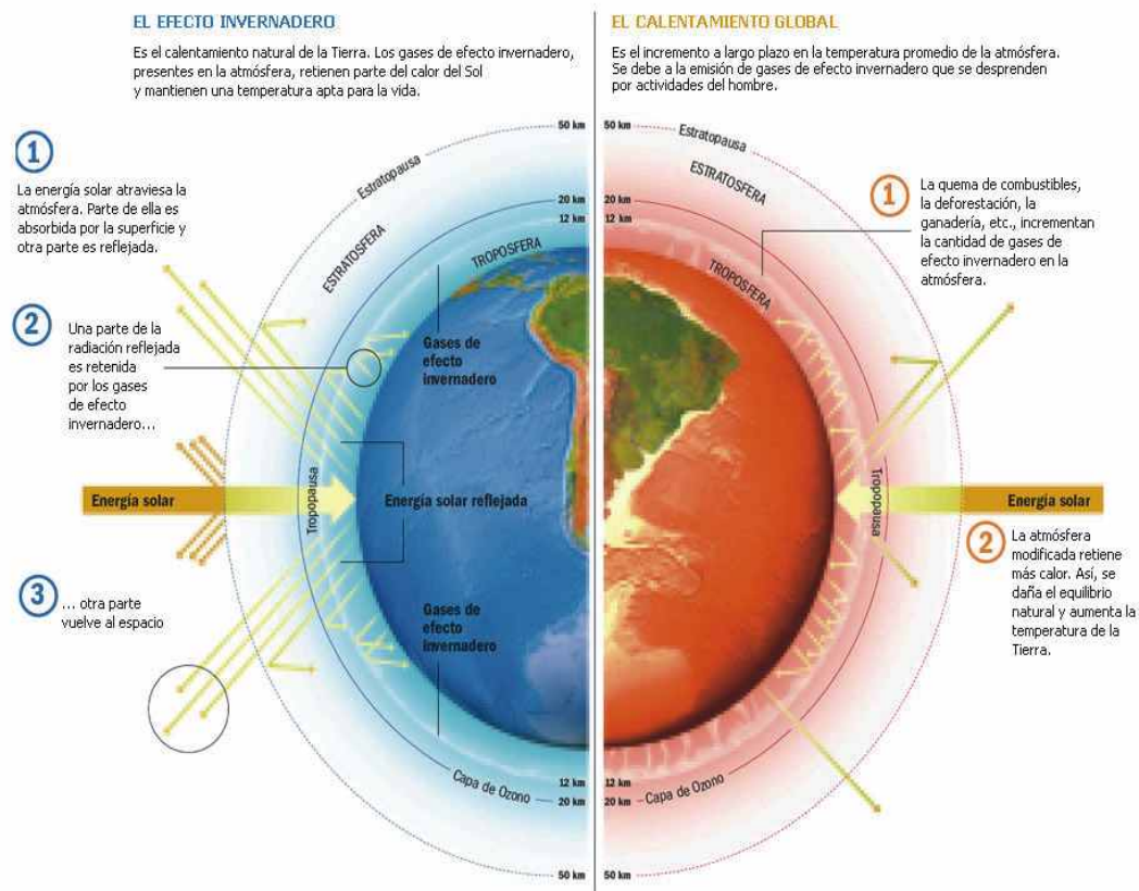
Fig. 2.1.- Calentamiento Global
